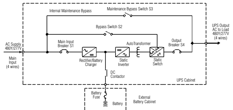
30 kVA (4 x 4)
